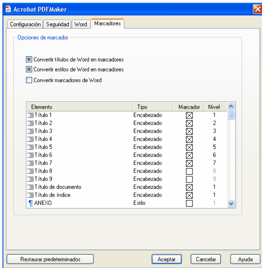
Figura 21. Configuración de Acrobat PDFMaker para la creación de marcadores.
